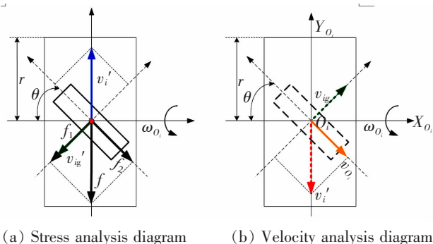
图1 A麦轮运动学分析
