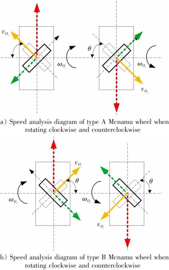
图 3 A 麦轮和 B 麦轮速度分析
