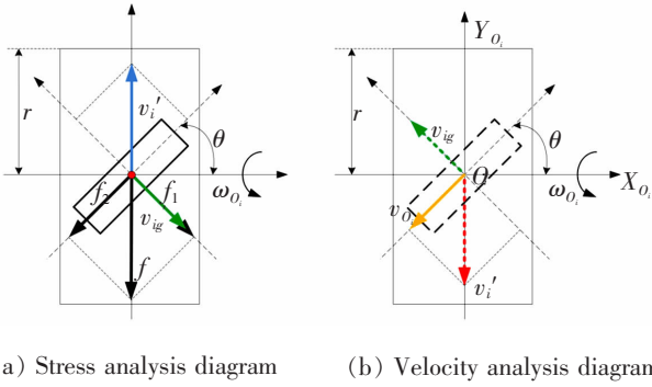
图 2 B 麦轮运动学分析
