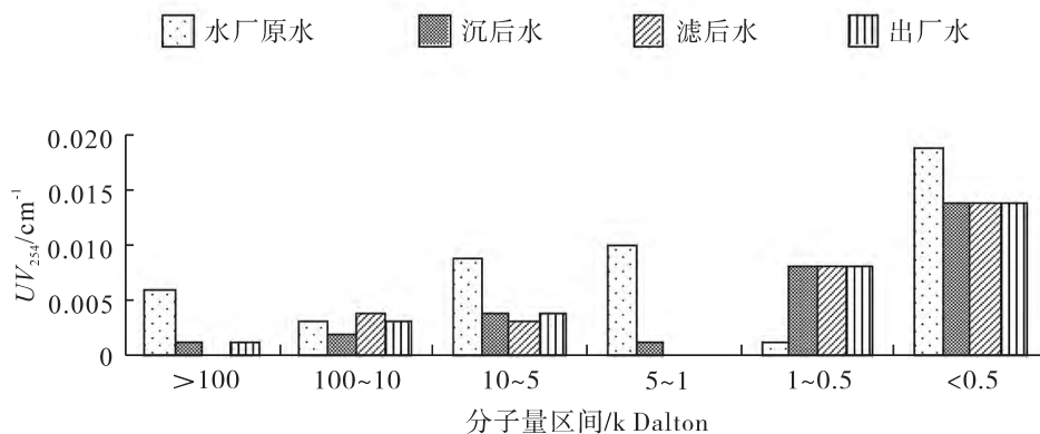
图5 各分子量区间 UV_{254} 变化
