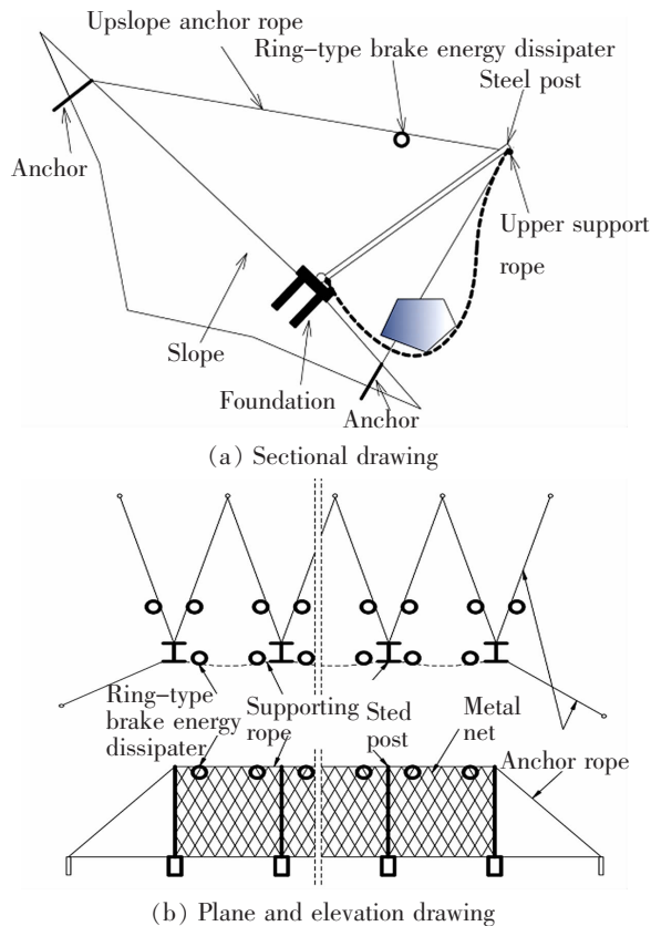
图2 被动柔性防护系统的组成
