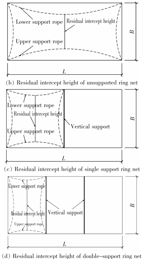
图1 缓冲距离与残余拦截高度示意图
