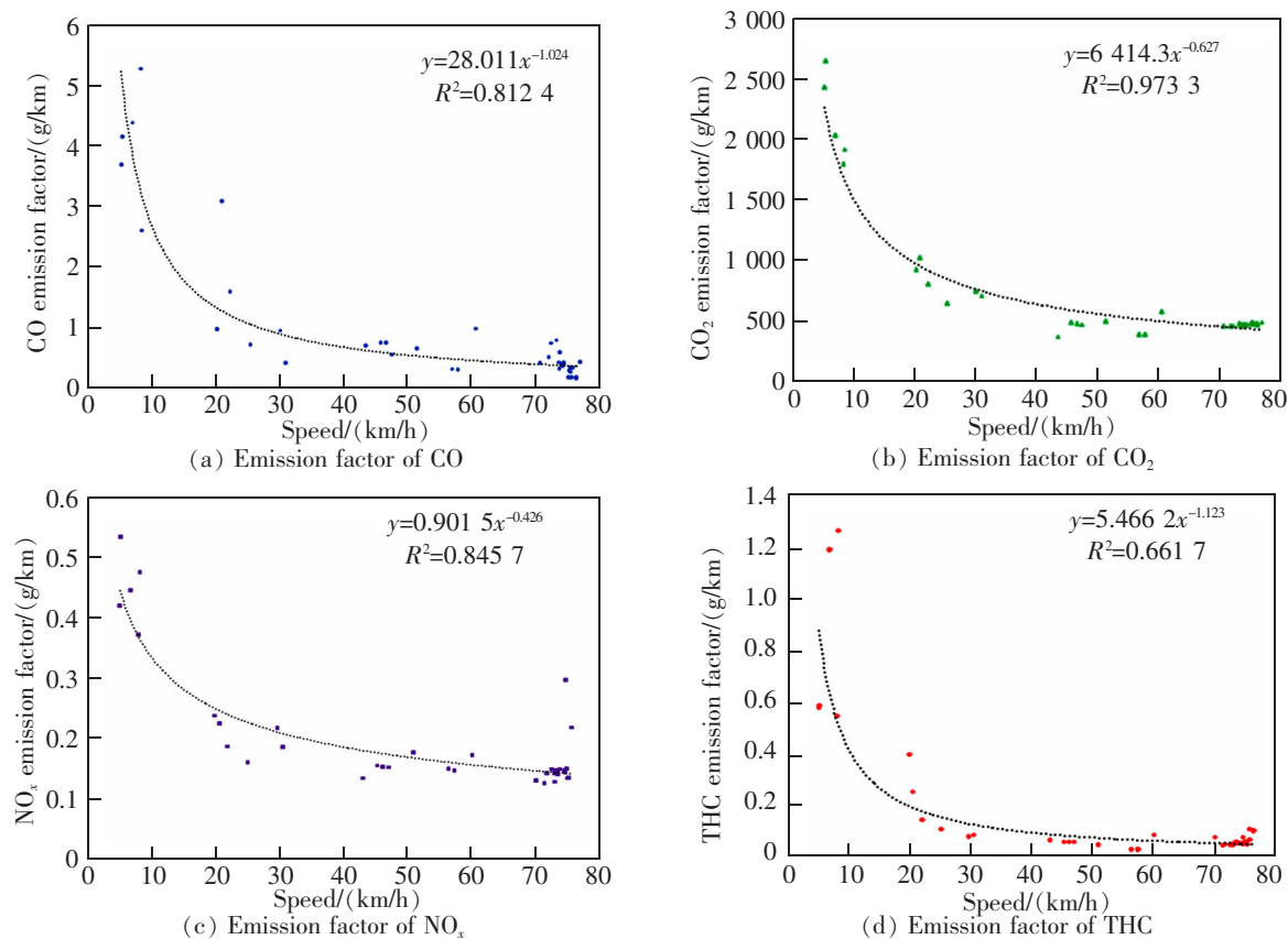
图6 车速对污染物排放的影响
