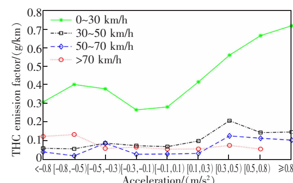
(d) Emission factor of THC
