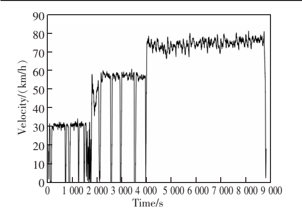
图 1 速度分布图 Fig.1 Velocity profile
