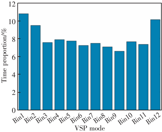
图 3 VSP 区间时间占比
