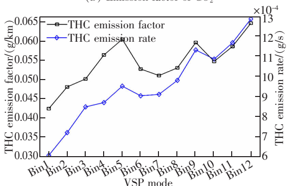
(d) Emission factor of THC
