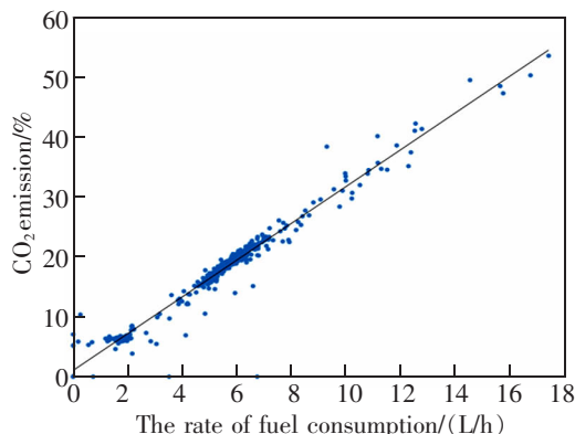
图 2 CO 2 浓度与燃油消耗率数据相关性
