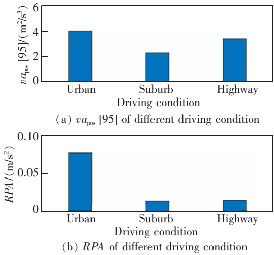
图 4 各路段行驶动力学参数
