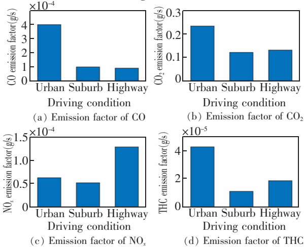
图 5 不同路段污染物排放因子
