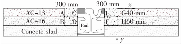
图 8 受力分析点示意图
