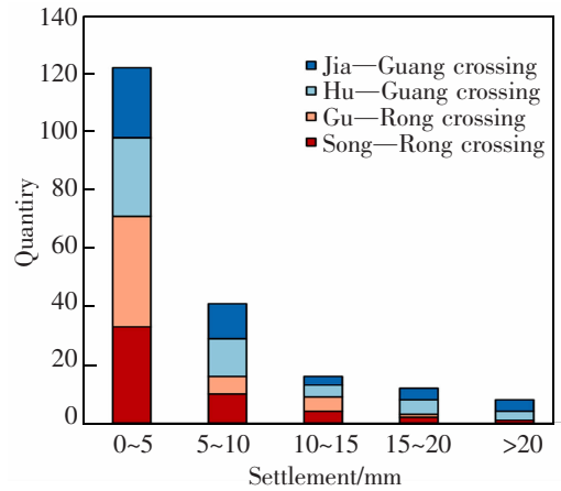
图4 过渡区路面沉降量分布情况
