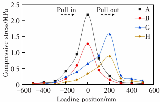
图 10 不同荷载作用位置下过渡区压应力分布图
