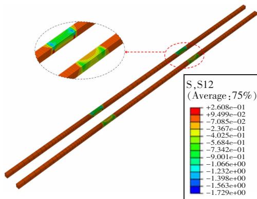
图 11 过渡区最大剪应力云图
