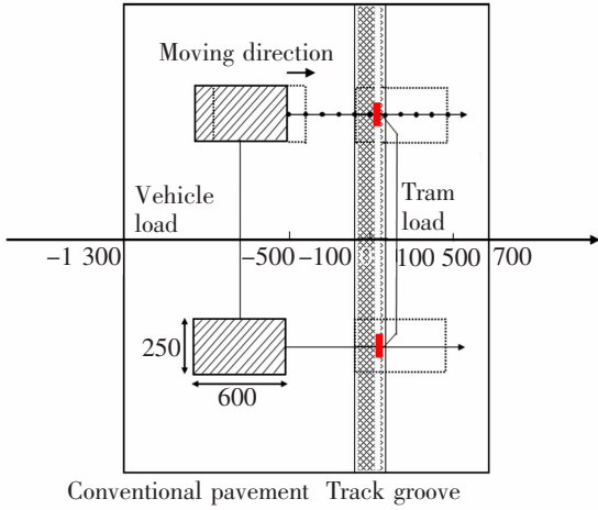
图 7 车辆荷载作用位置示意图(单位:mm) Fig.7 Schematic diagram of vehicle loading position (Unit:mm)
