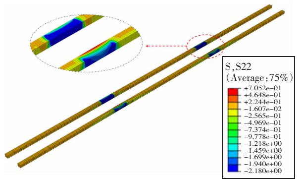
图 9 过渡区最大压应力云图
