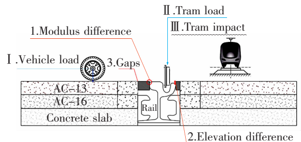
图5 路-轨过渡区结构和荷载特性
