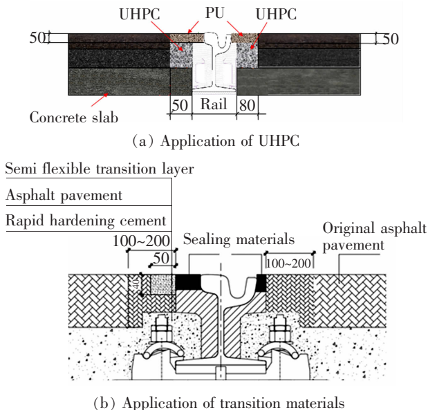
图 13 病害处治方案示意图(单位:mm)
