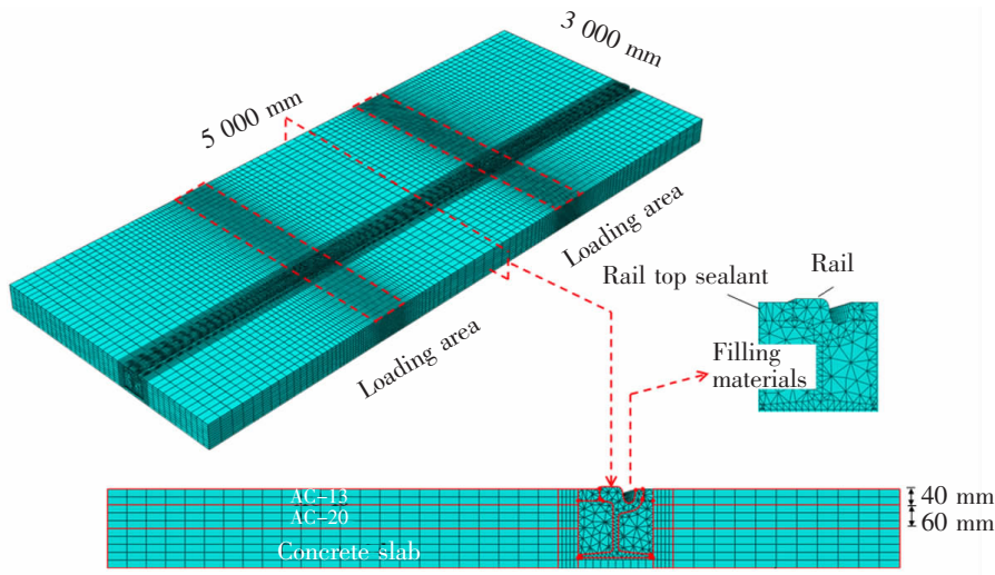
图 6 路-轨过渡区有限元分析模型
