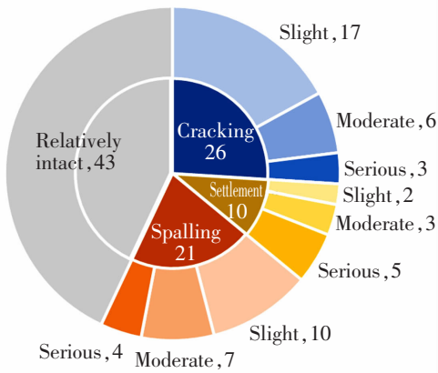
图2 过渡区病害类型分布图
