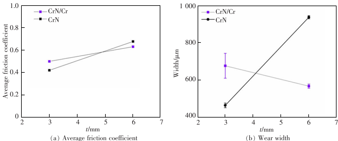
图 8 300 r/min、10 N 载荷下不同半径下平均摩擦系数与磨损宽度
