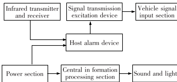
图 3 红外线报警装置结构图
