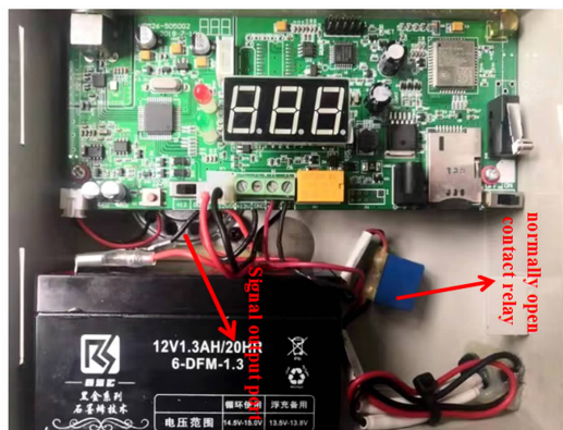
图 6 信号传输激发装置示意图
