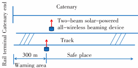
图 4 红外线发射、接收部分设置图
