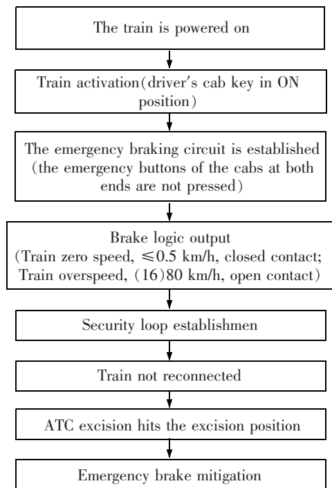
图1 紧急制动电路的建立
