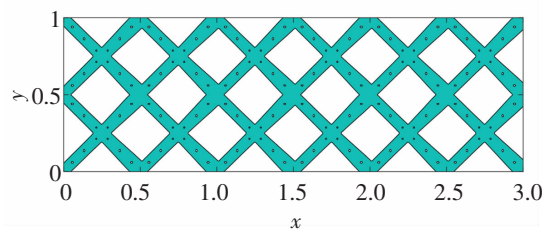
图 4 MBB 梁算例初始设计 ( a=0.1, G=0.1 )
