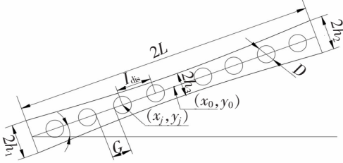
图1 微胶囊中心点坐标说明
