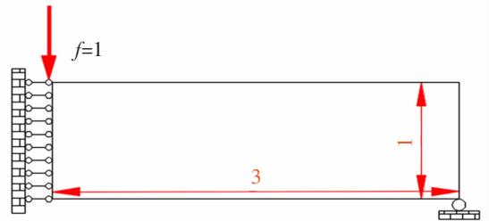
图 3 MBB 梁一侧设计域
