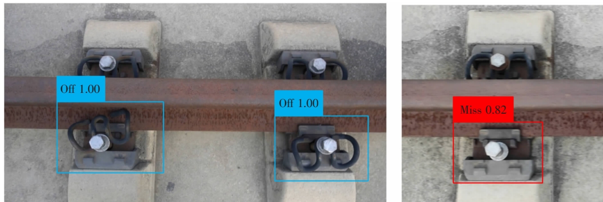
图 7 高铁扣件检测实例
