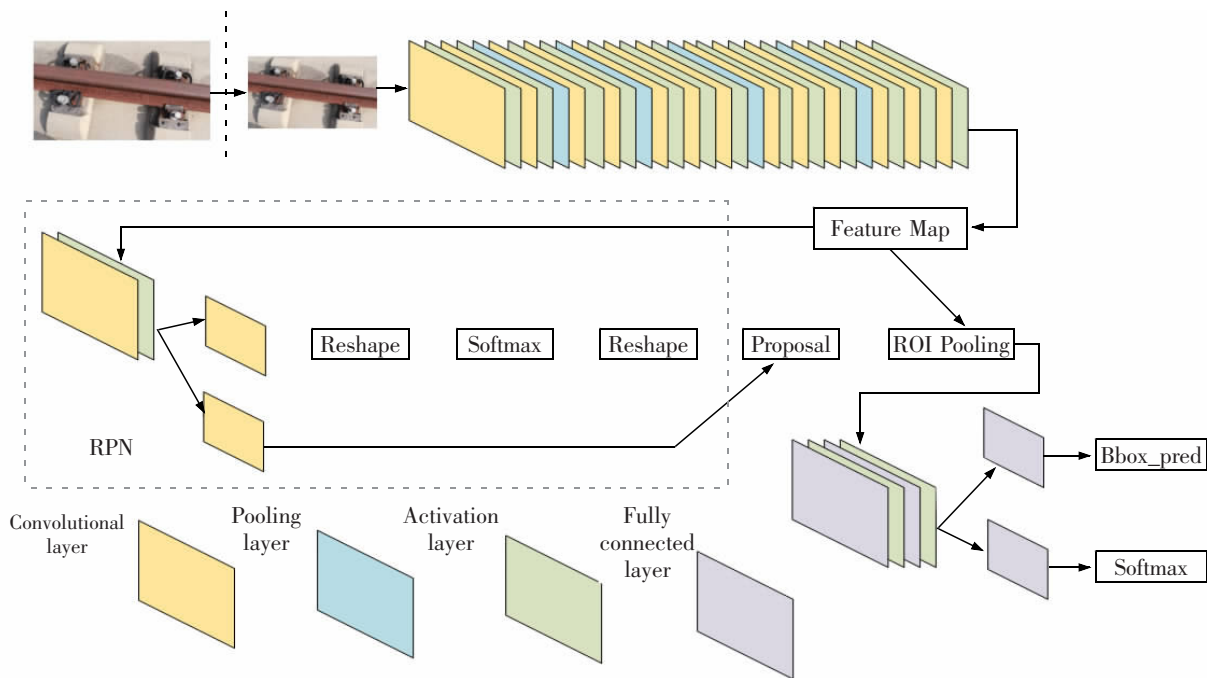
图1 Faster R-CNN 的网络结构图
