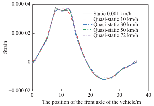
图12 第一跨跨中应变
