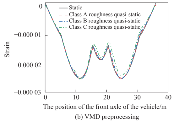
图9 桥墩支点应变
