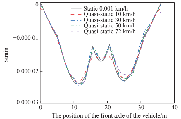
图14 桥墩支点应变
