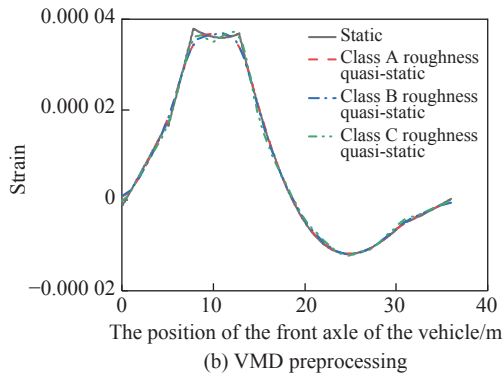
图7 第一跨跨中应变
