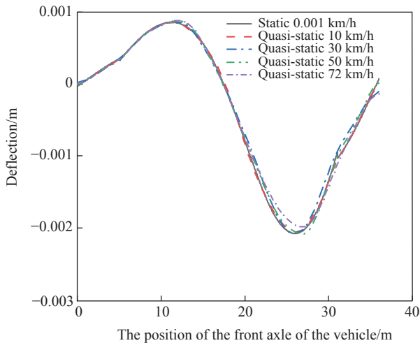
图11 第二跨跨中挠度
