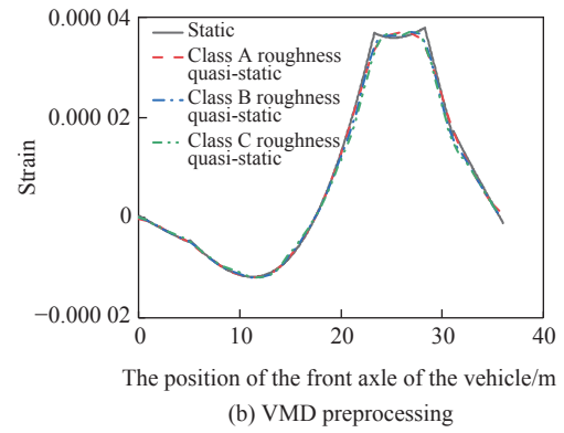
图8 第二跨跨中应变
