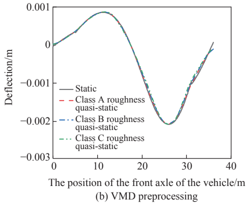
图6 第二跨跨中挠度
