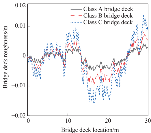
图4 桥面粗糙度模拟
