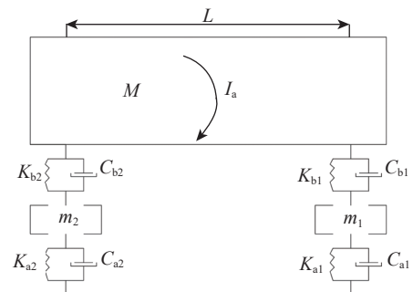
图3 双轴半车动力学模型
