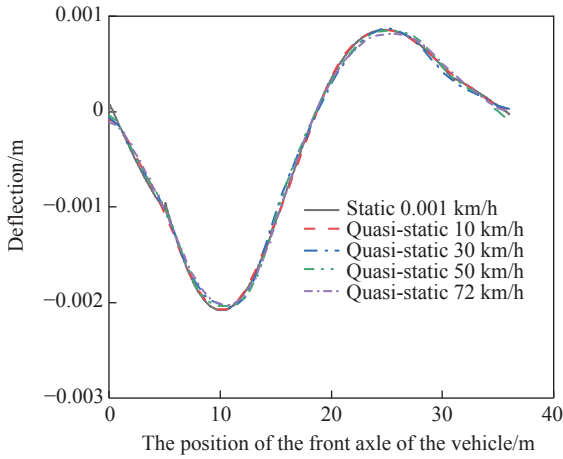
图10 第一跨跨中挠度
