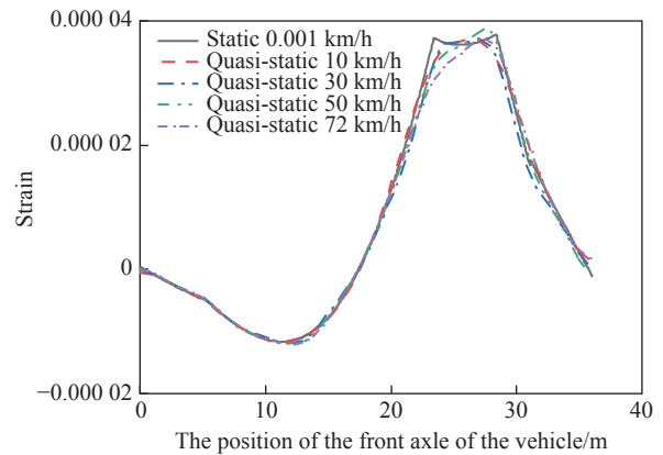
图13 第二跨跨中应变
