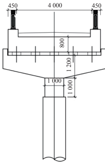
图1 桥梁横断面图(单位:mm)
