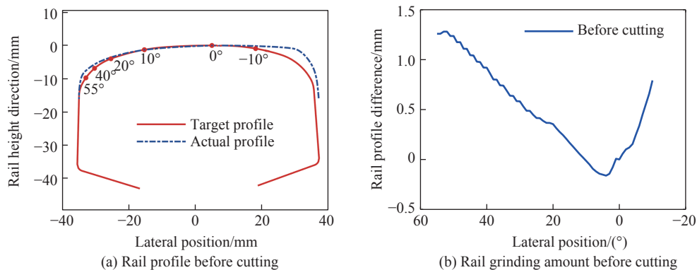
图6 切削前的钢轨廓形及钢轨打磨量曲线
