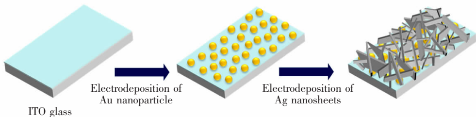
图1 Ag纳米片组装膜制备示意图
