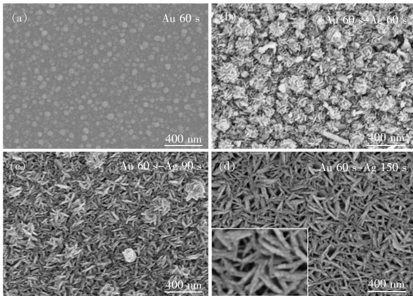
图 2 样品的 SEM 图片 (a) 为 Au 纳米颗粒; (b), (c), (d) 为分级 Ag 纳米片组装膜, 电化学沉积时间分别 60, 90, 150 s Fig. 2 SEM images of (a) Au nanoparticles; (b), (c), (d) hierarchical Ag nanosheet-assembled films electrodeposited for 60 s, 90 s, 150 s
