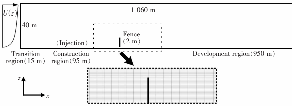
图 2 CFD 模拟计算域与局部网格示意
