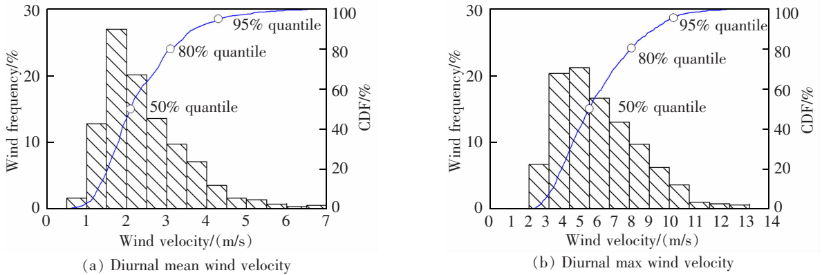
图 1 日均风速的风频与累计分布函数
