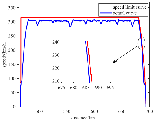
图5 动车组实际运行“V-S”曲线
