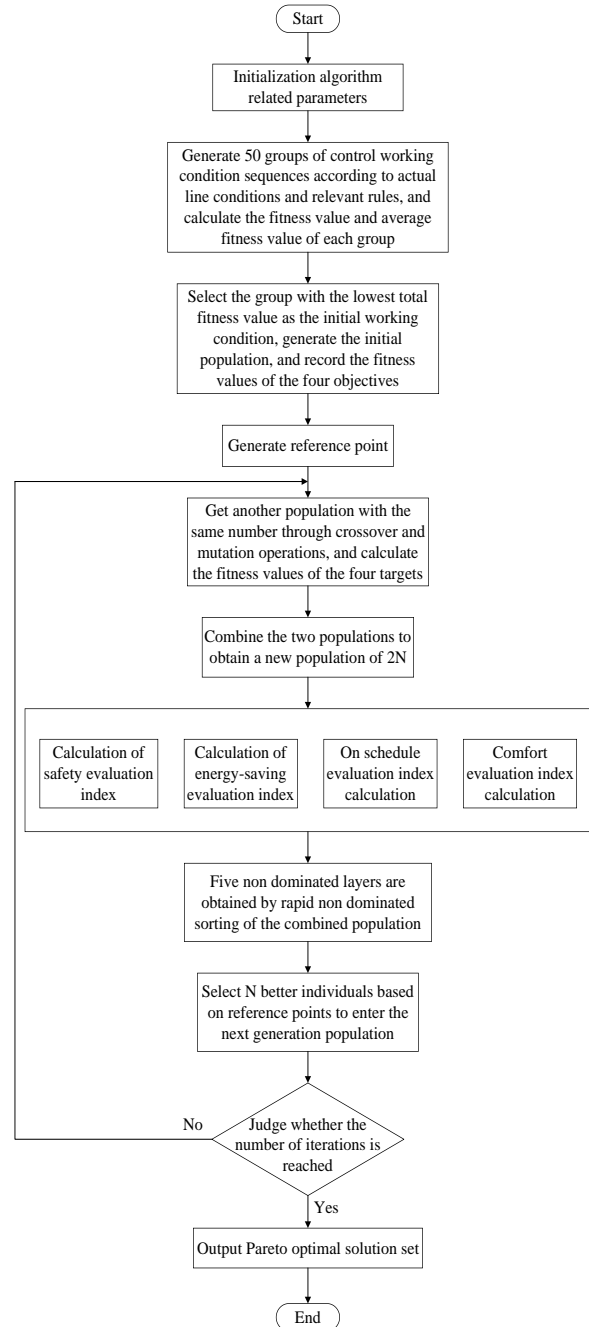
图4 高速列车多目标优化算法流程图
