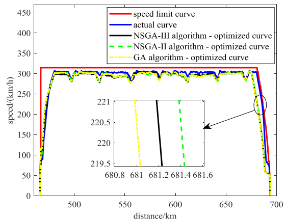
图10 不同算法对比的运行“V-S”曲线
