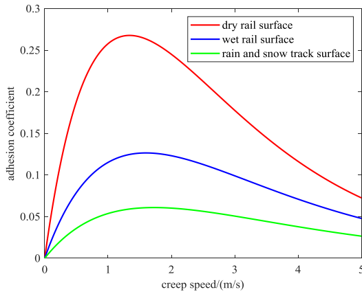
图3 不同轨面黏着特性曲线
