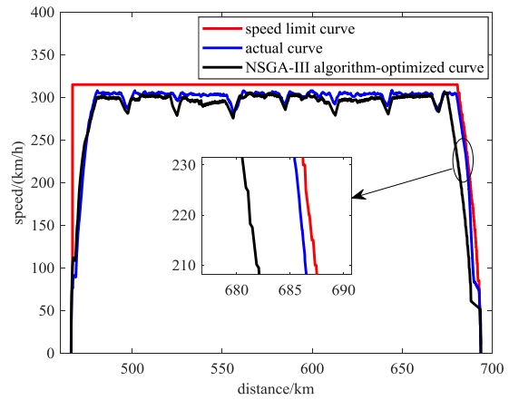
图6 动车组优化后的运行“V-S”曲线
