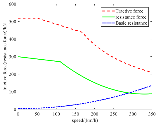
图1 CRH380AL型列车牵引/制动特性曲线
