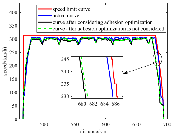
图8 不同模型对比的运行“V-S”曲线
