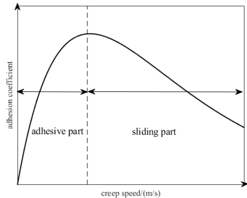
图2 列车运行中的轮轨黏着曲线
