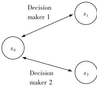
图1 可行状态单边转移图
