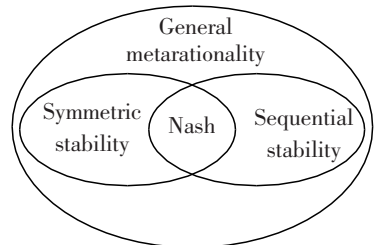
图2 4种稳定性类型的相对关系
