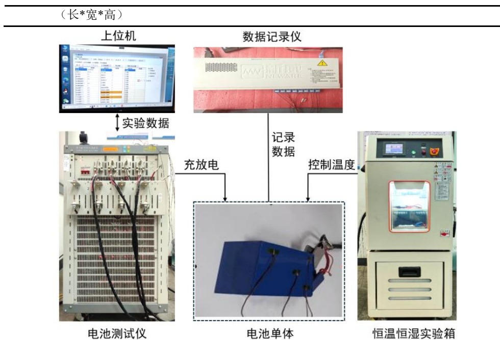
图 6 实验平台
