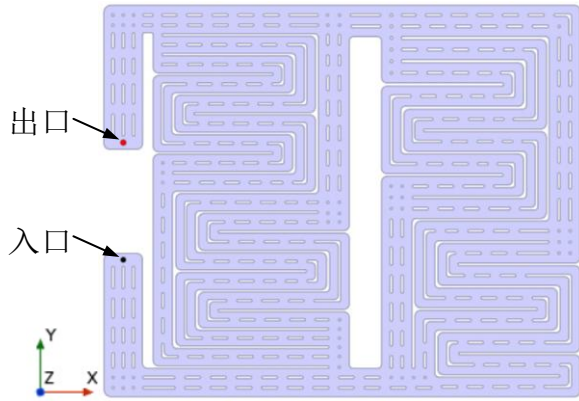
图 2 液冷板几何模型
