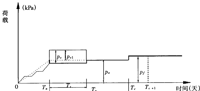
图 1 考虑超载和轨道列车荷载简化加载示意图
