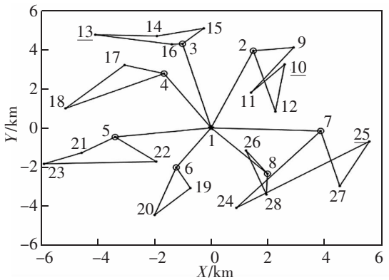
图 6 改进算法求解的路径优化结果
