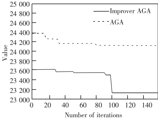
图 5 迭代结果对比图
