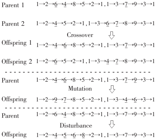
图 2 子路径交叉变异扰动
