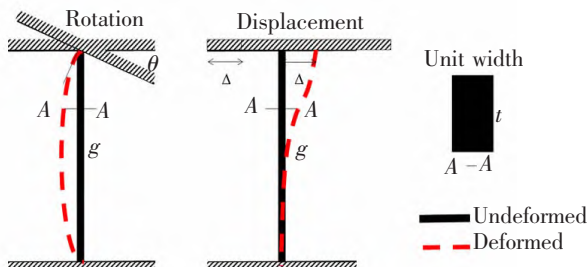
图 6 简化模型 Fig.6 Simplified model
