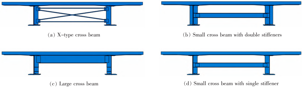
图3 主梁结构形式
