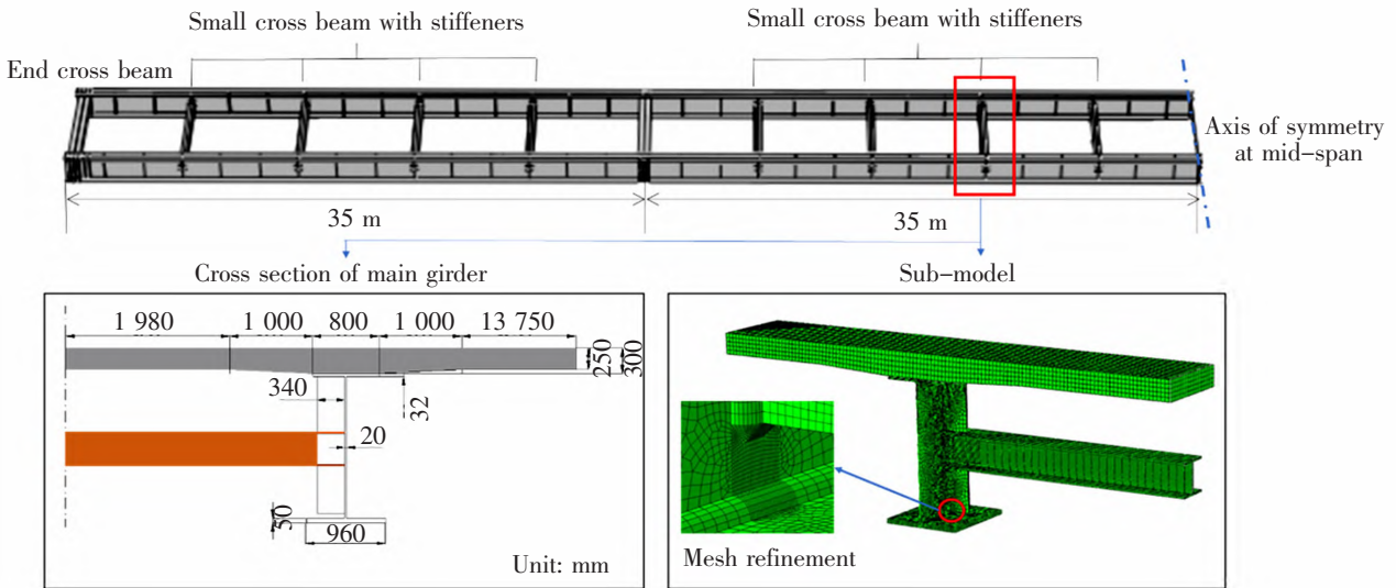
图 1 有限元模型
