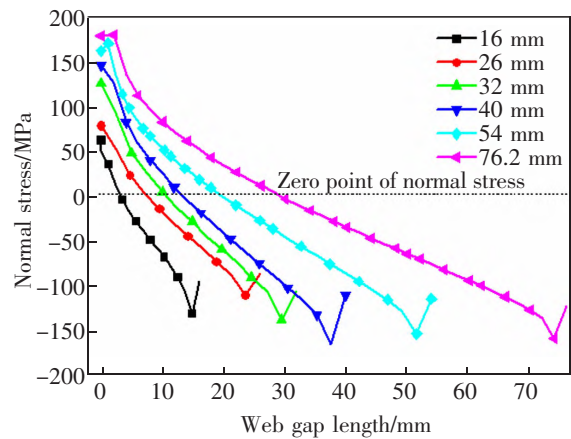
图 9 腹板间隙表面正应力
