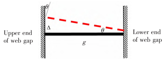
图 7 转角与位移的关系
