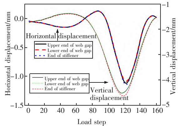
图5 位移变化
