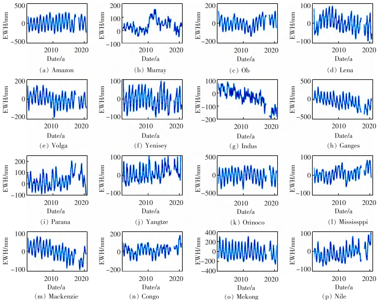
图1 全球典型流域等效水高变化
