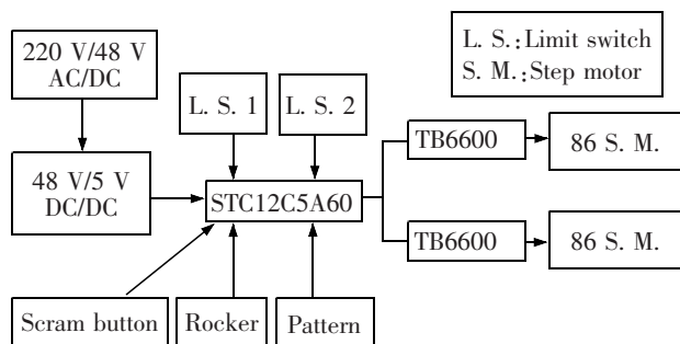
图 8 控制框图
