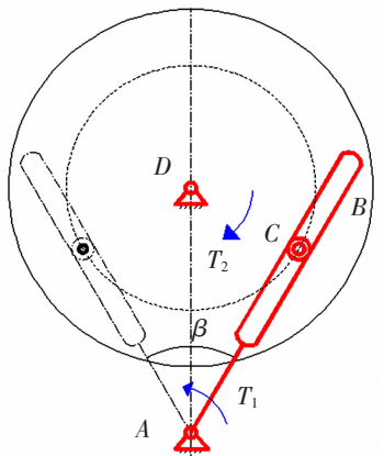
图 5 从整周转动到往复摆动的变换 Fig.5 Transformation from revolution to rock
