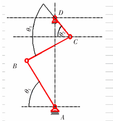
图 3 四杆机构简图
