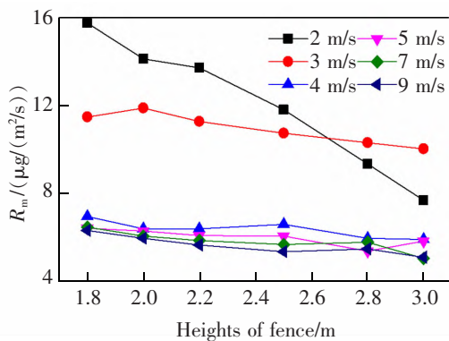
图 6 不同围挡高度和来流风速下离围挡 42 m 的平均扬尘排放率
