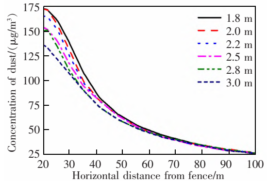
图 4 不同围挡高度下 1.5 m 呼吸高度处扬尘浓度水平扩散结果—来流风速 2 m/s
