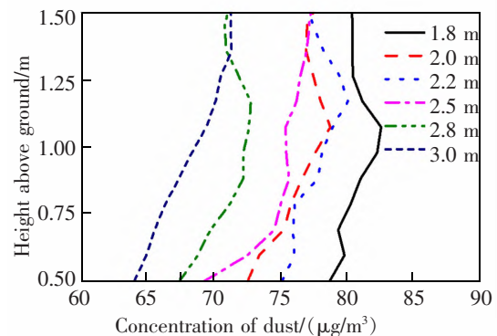
图 5 不同围挡高度下离围挡水平长度 42 m 处扬尘浓度竖向扩散结果—来流风速 2 m/s
