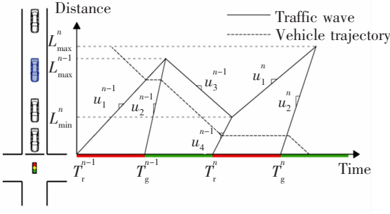
图 7 周期存在二次排队的网联车
