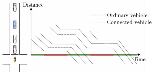
图 4 过饱和交叉口车辆轨迹
