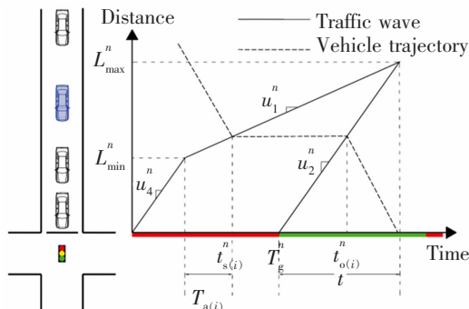
图 5 排队过程示意图
