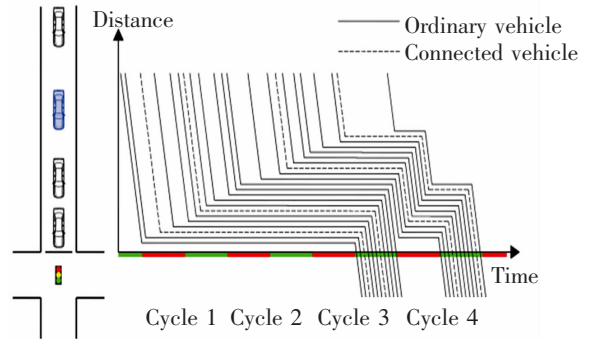
图 8 溢出回流期间的车辆轨迹
