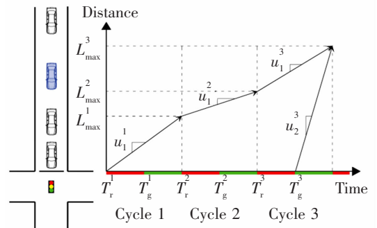
图 9 溢出回流期间交通冲击波示意图
