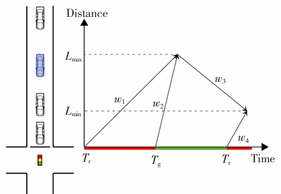
图3 冲击波产生原理及传播过程
