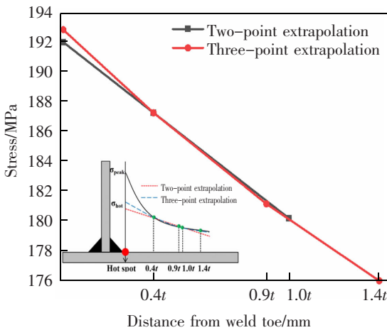
图 15 热点应力外推结果 ( t=16\text{ mm} )
