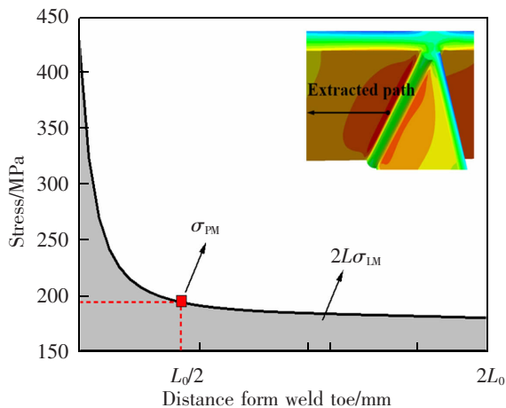
图 17 特征应力的确定
