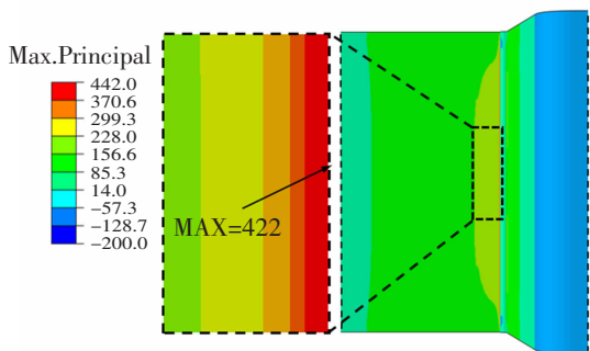
图 11 模拟轮载下焊趾附近应力分布(单位:MPa)
