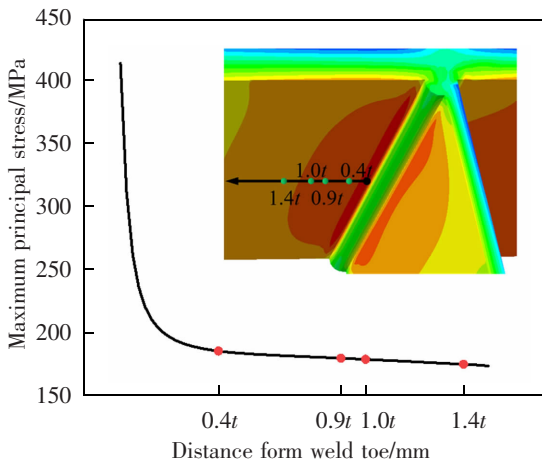
图 14 外推点最大主应力
