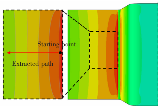
图7 应力提取路径
