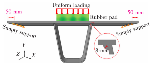
图5 模型荷载及边界(单位:mm)
