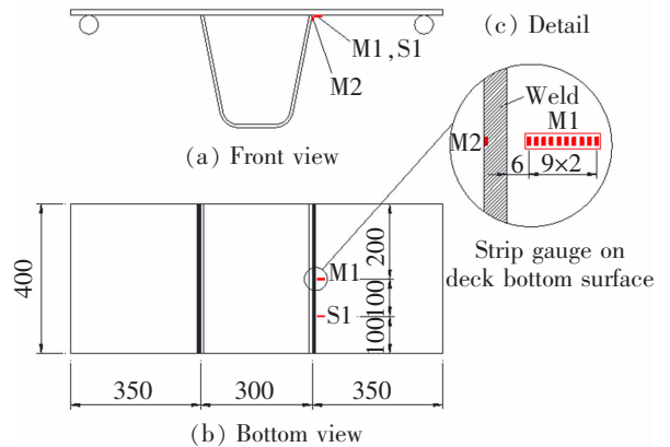
图 9 RD 试件测点布置(单位:mm)
