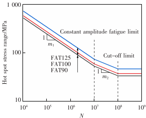
图 16 热点应力 S-N 曲线
