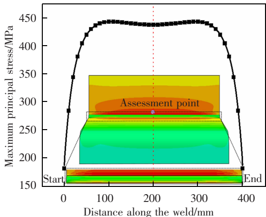
图 13 沿焊缝最大主应力分布
