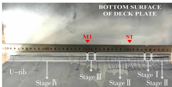
图 12 RD 节点疲劳开裂过程
