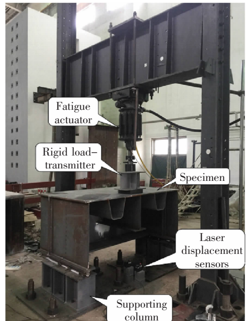
图4 RD试件加载装置
