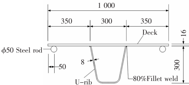
图3 RD节点构造尺寸(单位:mm)
