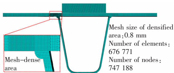
图6 模型网格划分及加密区
