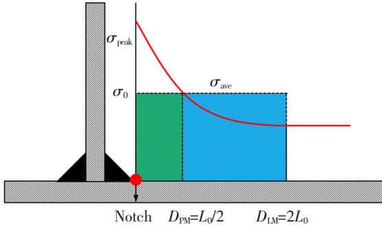
图2 点法与线法示意图
