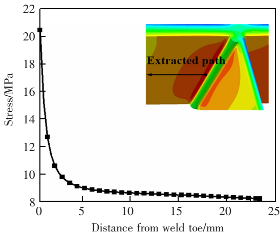
图 8 提取路径上的应力
