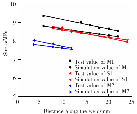
图 10 各测点应力实测值与模拟值对比
