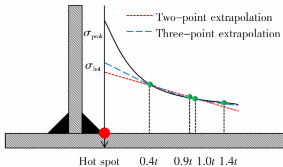
图 1 热点应力外推示意图
