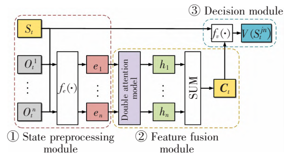
图 2 状态价值网络
