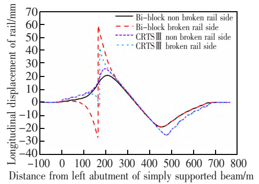
图 13 钢轨纵向位移
