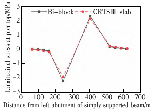
图 5 墩顶纵向力
