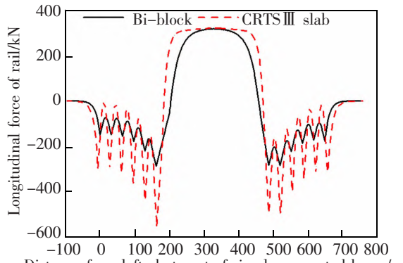
图 3 钢轨纵向力
