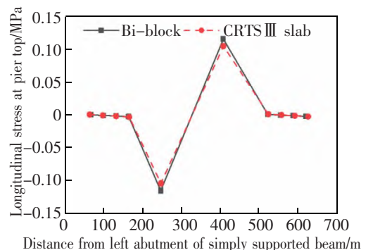
图 8 墩顶纵向力
