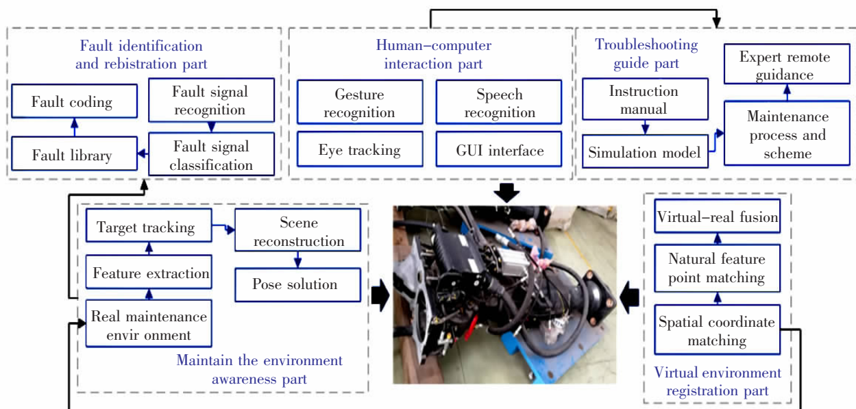
图 1 基于混合现实的动车组车钩辅助检修系统技术框架
