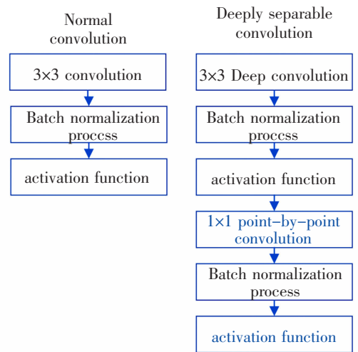
图3 全卷积与深度可分离卷积的结构
