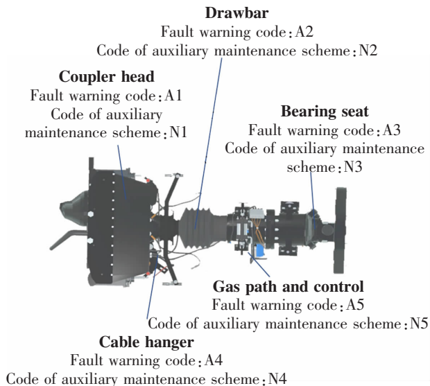
图6 车钩特征划分及故障编号示意图
