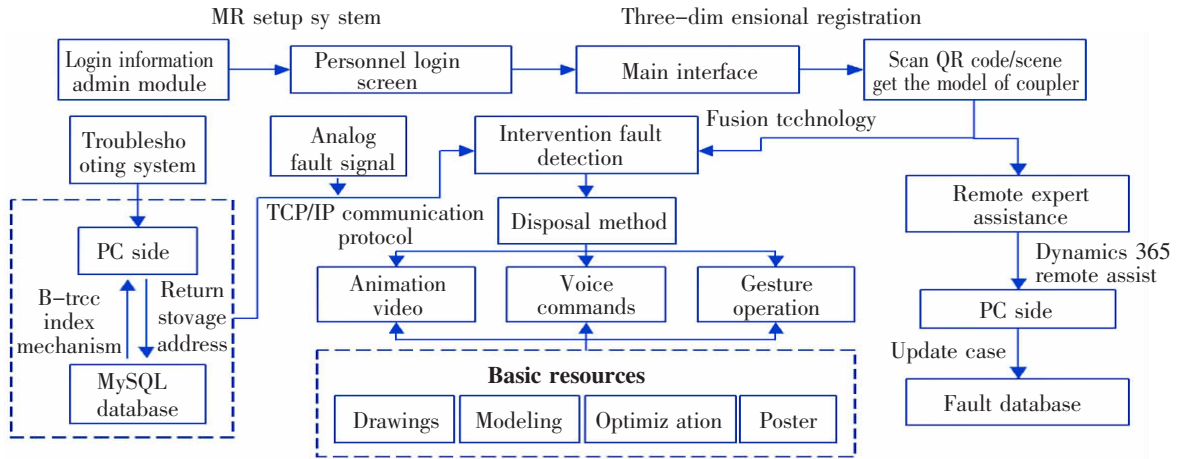
图2 系统开发技术路线图
