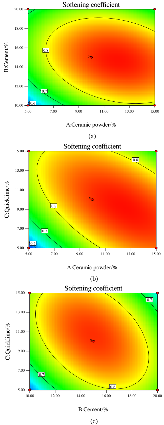
图 2 两因素交互作用对软化系数的影响等高曲线图
