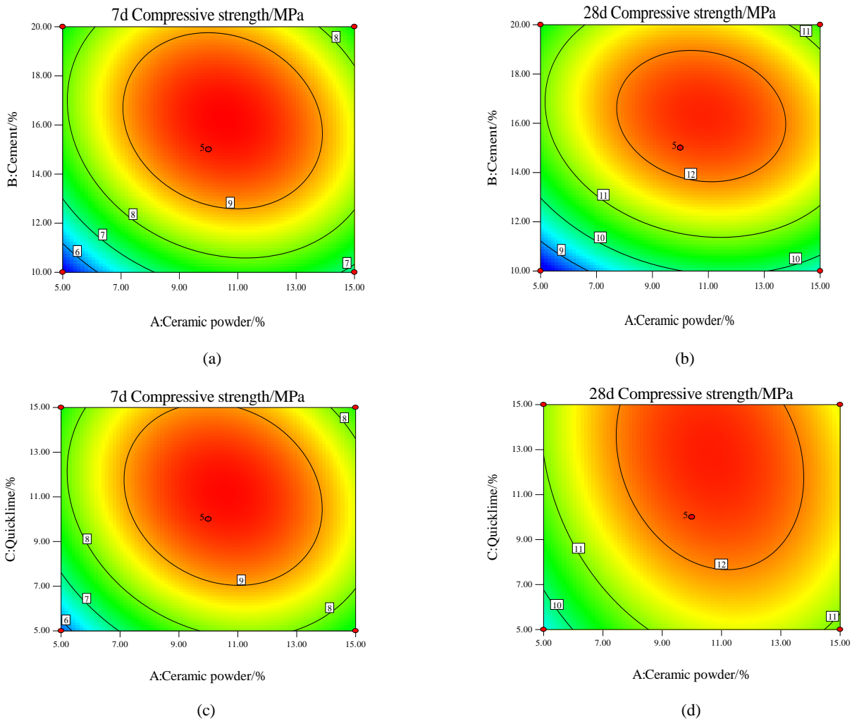
图 1 两因素交互作用对抗压强度的影响等高曲线图
