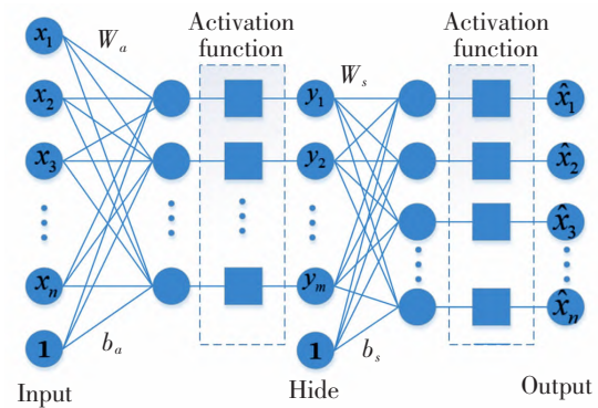
图1 AE网络结构图
