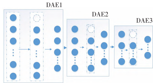
图 4 SDAE 网络结构图 Fig.4 SDAE network
