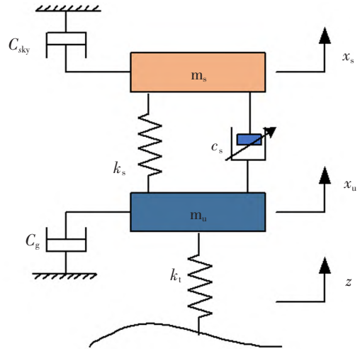
图7 理想混合天地棚控制模型
