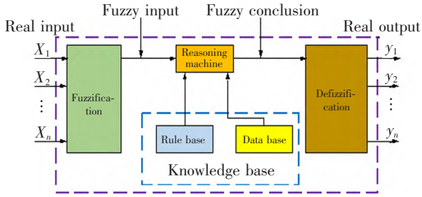
图6 模糊控制原理
