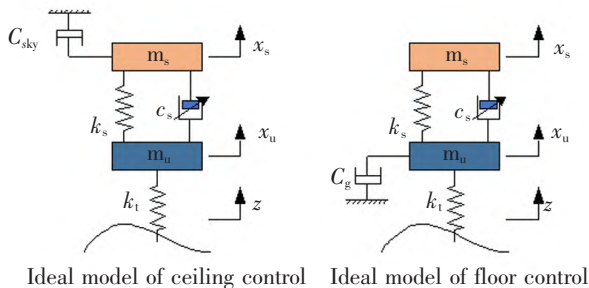
图5 天棚和地棚理想模型
