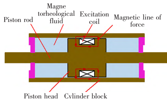
图4 磁流变阻尼器结构示意图
