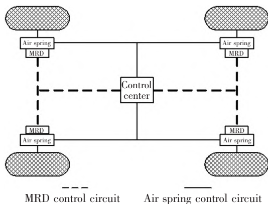
图2 磁流变半主动空气悬架控制示意图
