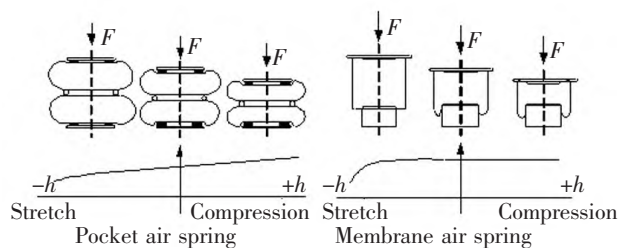
图3 空气弹簧工作原理示意图
