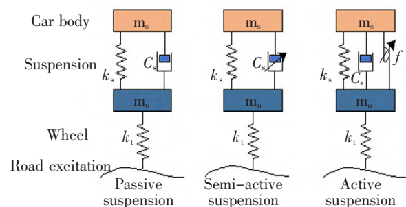
图 1 各类悬架结构示意图
