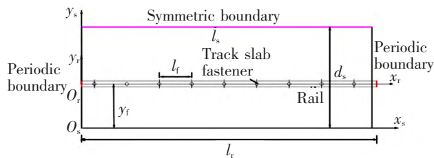
图 1 一个橡胶浮置板轨道胞元计算图 Fig.1 Computational diagram of a rubber floating plate track cell element
