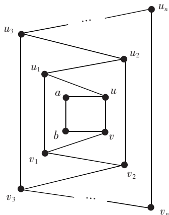
图2 第一型环己烷类图 G
