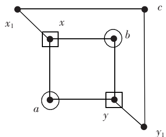
图7 图 M_0 的导出子图 H
