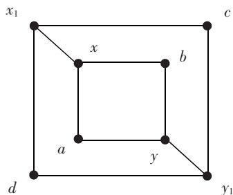
图6 图 M 的导出子图 M_0
