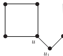
图 1 环己烷类图的 4-边形上只有一个 3 度点
