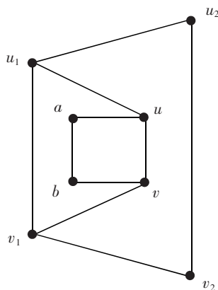
图3 G 图的导出子图 G_0
