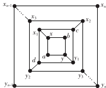
图5 第二型环己烷类图 M
