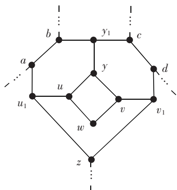
图8 第三型环己烷类图 N Fig.8 The type III cyclohexane graph N
