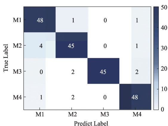
图6 DCA模型诊断结果混淆矩阵
