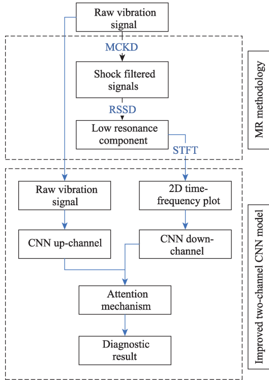
图1 诊断模型流程图
