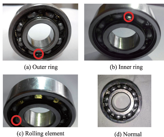
图3 4种状态滚动轴承
