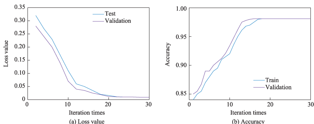
图5 DCA模型损失及准确率
