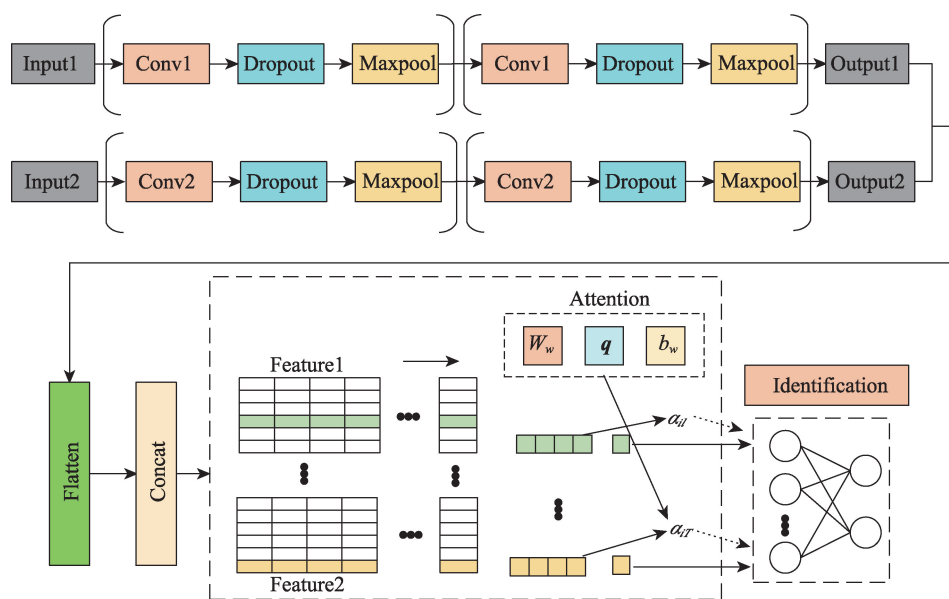
图2 DCA模型架构
