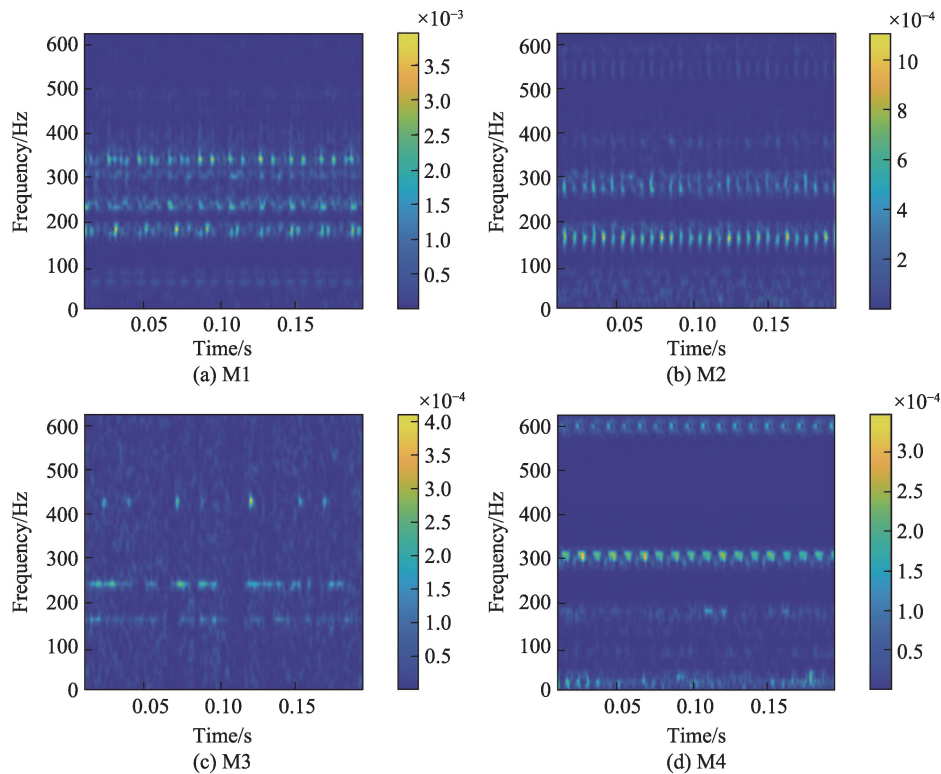
图4 MR方法处理结果时频图
