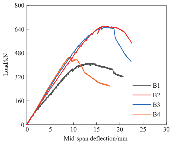
图4 荷载-跨中挠度曲线
