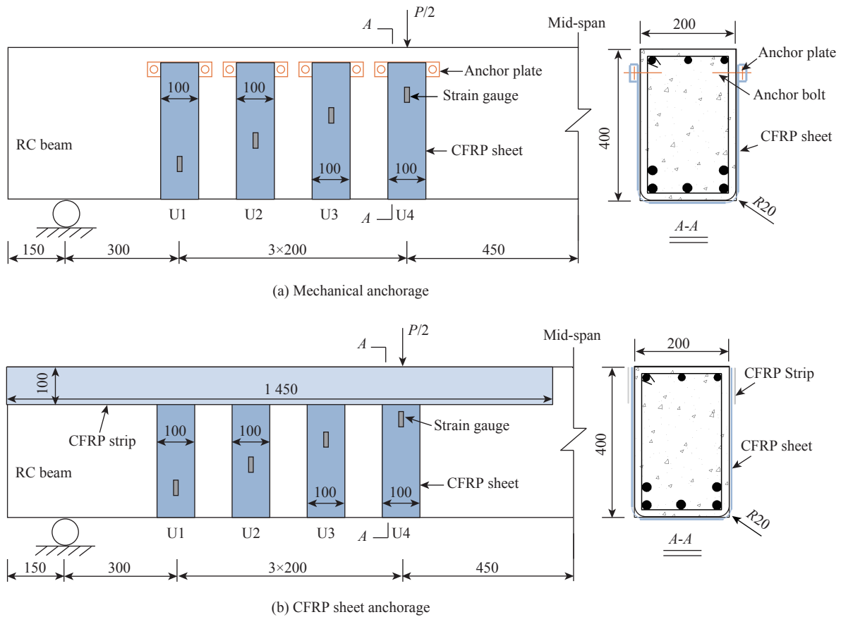
图2 加固方案及锚固方式(单位:mm)
