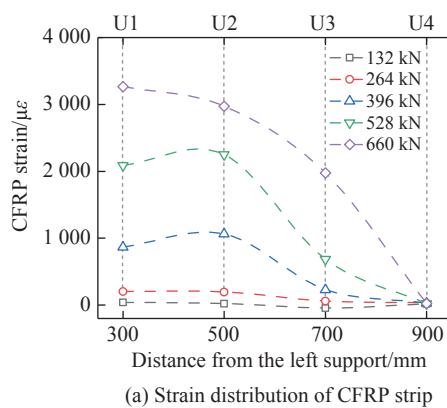
图5 试件B2中CFRP和箍筋的应变发展
