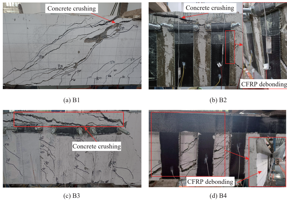
图3 试件的失效照片
