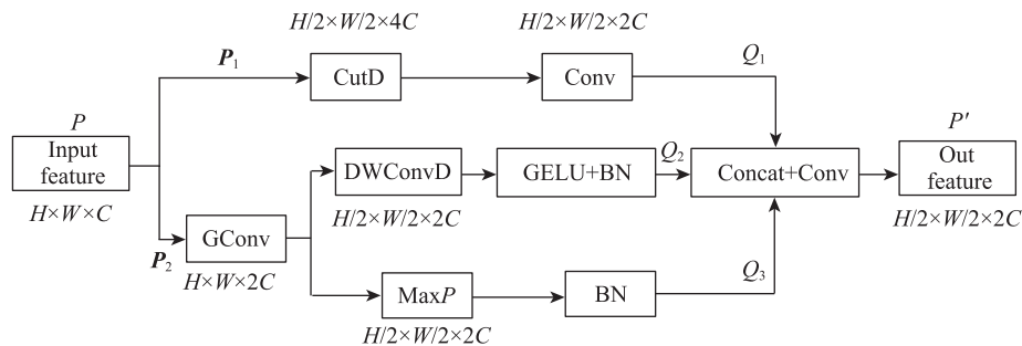
图2 下采样模块 IDM 结构图 Fig. 2 Structure diagram of IDM
