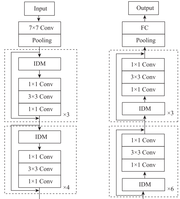
图1 改进 ResNet50 的网络结构示意图 Fig. 1 Diagram of the improved network structure of ResNet50
