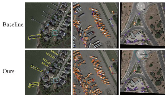
图5 在DOTA数据集上的可视化结果
