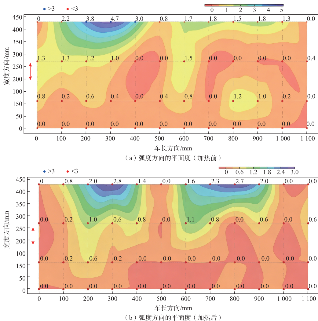
图5 车顶结构弧度方向的平面度变化
