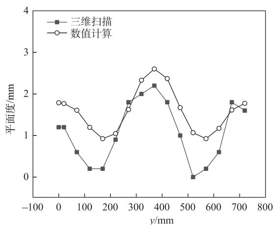
图18 测量点平面度对比( x=530 )
