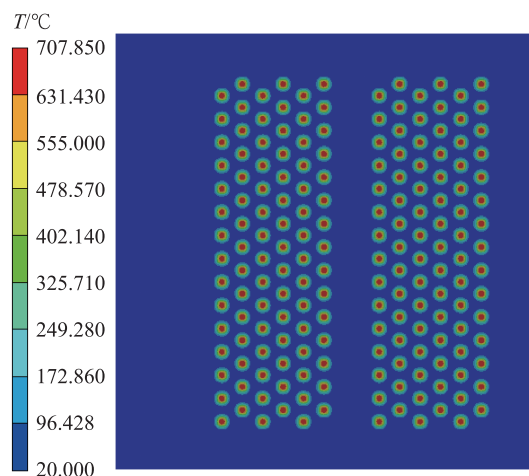
图15 侧墙结构表面温度分布图
