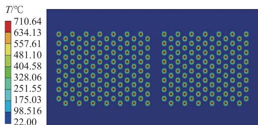
图8 车顶薄板结构温度分布图
