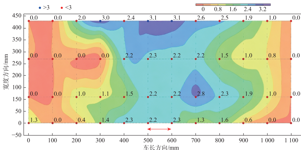
(b) 长度方向的平面度 (加热后)
