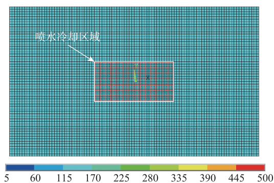
图2 薄板模型及喷水冷却区域
