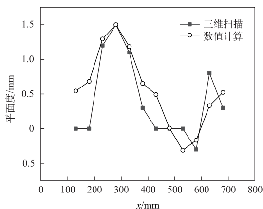
图19 测量点平面度对比( y=170 )
