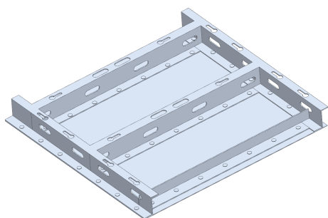
图13 侧墙结构三维模型
