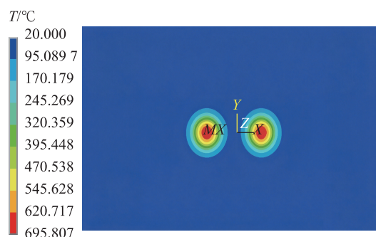
图4 小试板温度分布云图
