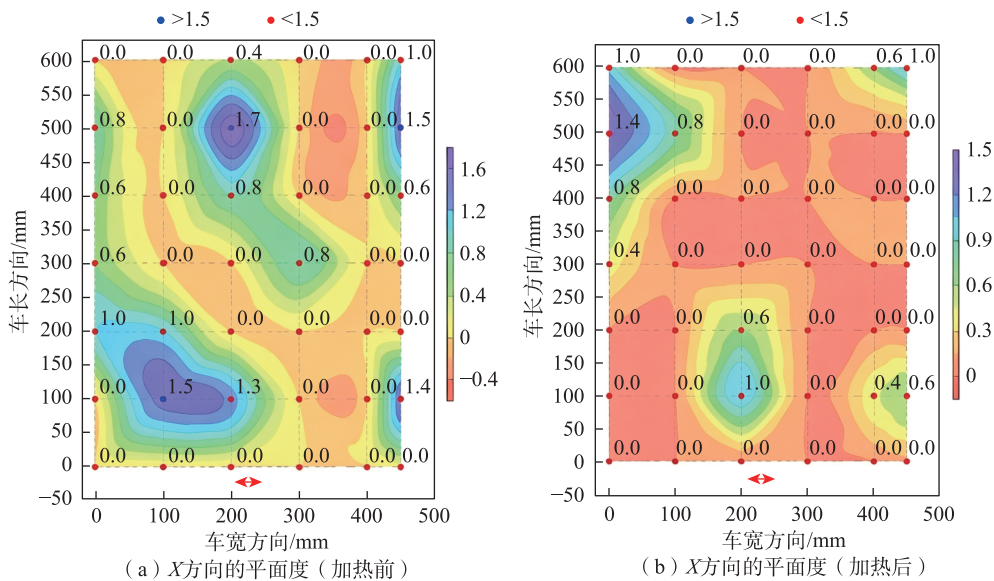
图11 侧墙结构X方向的平面度
