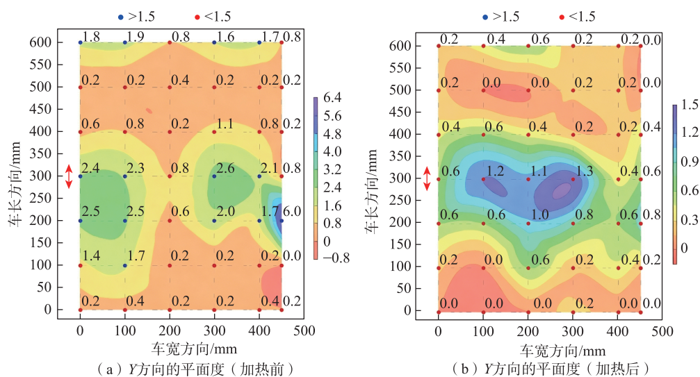
图12 侧墙结构Y方向的平面度
