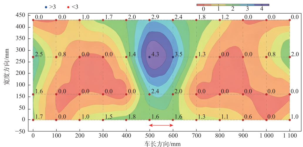
(a) 长度方向的平面度 (加热前)
