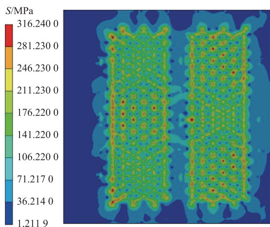
图17 薄板等效应力云图
