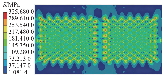
图10 薄板米塞斯应力云图
