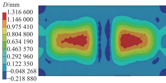
图9 车顶垂向位移云图
