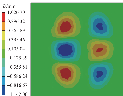
图16 垂向位移云图
