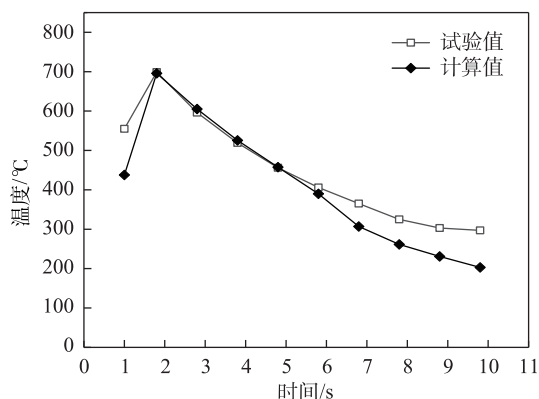
图3 A点温度变化曲线
