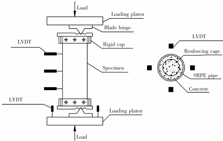
图 2 试验装置和测点布置
