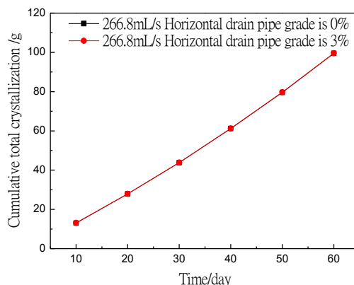
(d) 水流量为266.8mL/s时接头每延米结晶累积量数据
