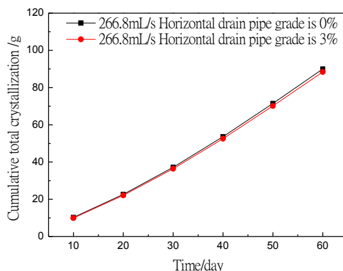
(e) 水流量为266.8mL/s时横向排水出口每延米结晶累积量数据
