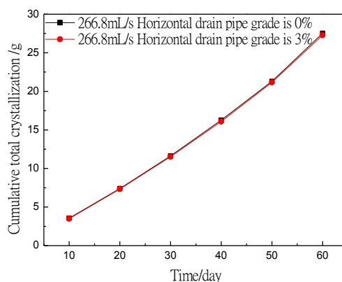
(a) 水流量为266.8mL/s时环向排水管每延米结晶累积量数据
