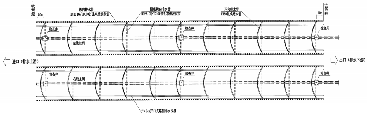
图 1 排水系统
