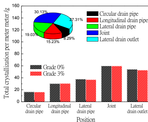
(c) 水流量为133.4mL/s时隧道各部分每延米结晶量数据
