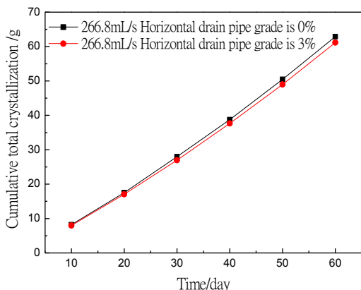
(c) 水流量为266.8mL/s时横向排水管每延米结晶累积量数据
