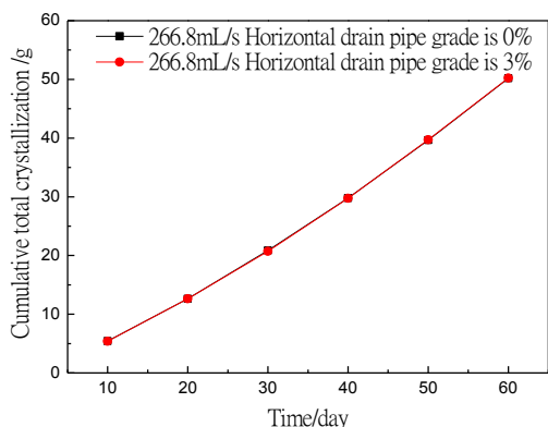
(b) 水流量为266.8mL/s时纵向排水管每延米结晶累积量数据
