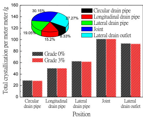
(a) 水流量为266.8mL/s时隧道各部分每延米结晶量数据
