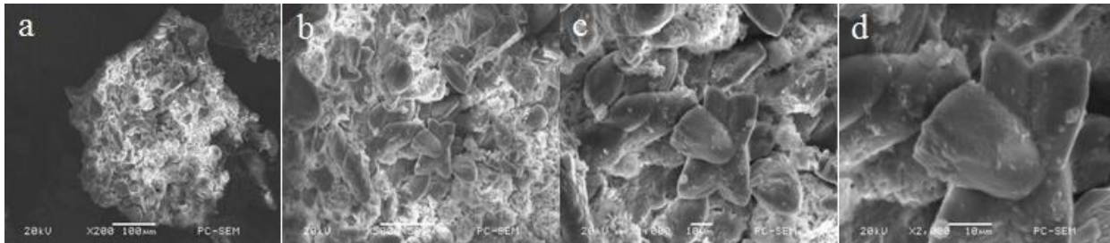
图3 SEM电镜扫描((a)200倍,(b)500倍,(c)1000倍,(d)2000倍)
