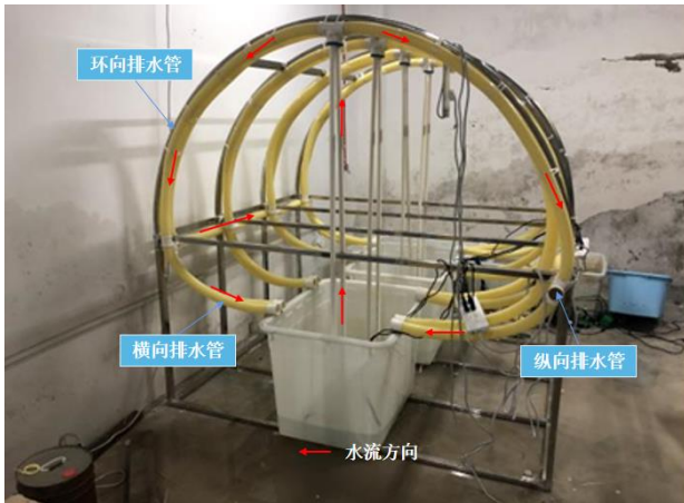
图 2 实验装置
