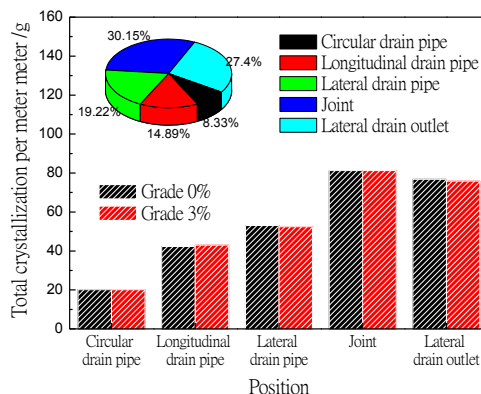
(b) 水流量为200.1mL/s时隧道各部分每延米结晶量数据
