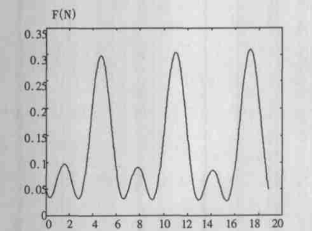
图6 垂直方向上的接触力 \theta(\text{rad})
