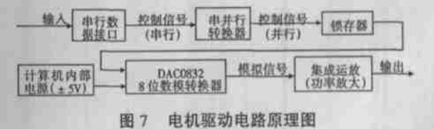
图7 电机驱动电路原理图
