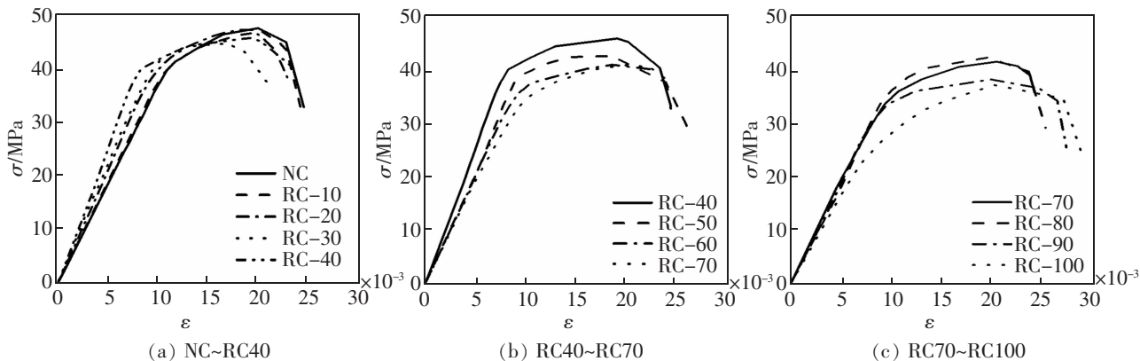
图4 不同取代率再生陶瓷粗骨料混凝土28 d的应力-应变全曲线
