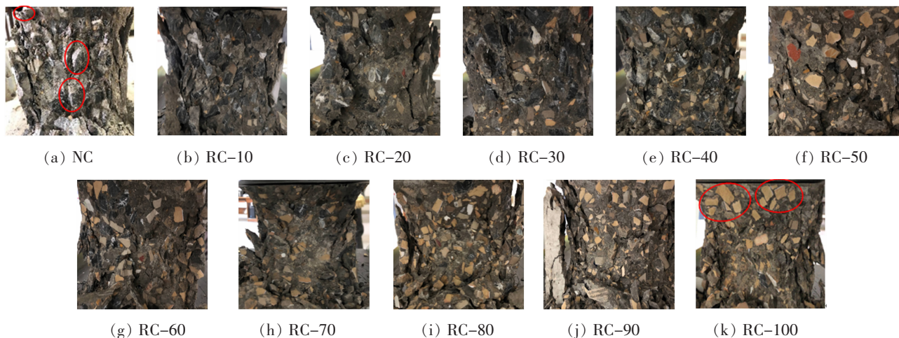
图 3 不同取代率再生陶瓷粗骨料混凝土试块 28 d 的破坏形态
