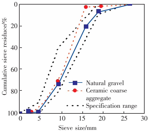
图2 粗骨料粒径分布
