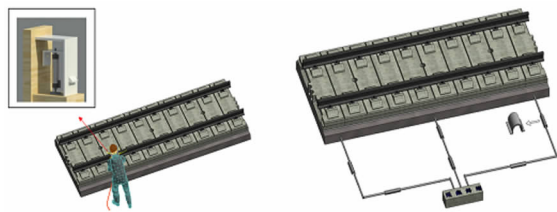
图6 安装流程模拟
