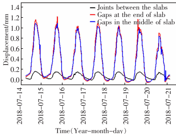
图 9 位移变化规律
