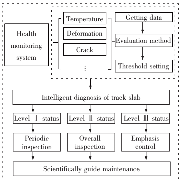
图 8 伤损预警方案
