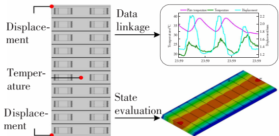
图 7 数据库与 BIM 模型联动方案
