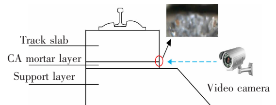
图 4 裂缝扩展监测示意图
