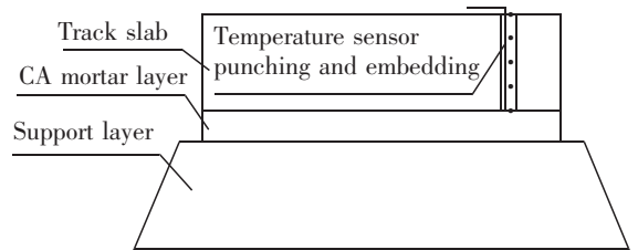
图 2 温度传感器布置图
