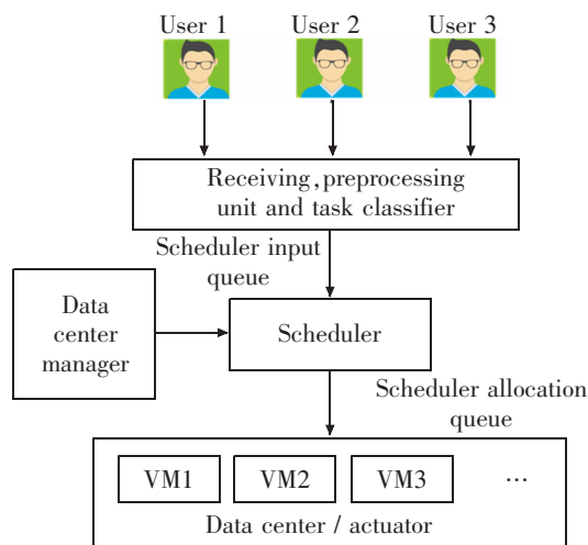
图 1 紧急任务动态调度模型
