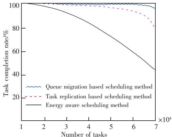
图 5 3 种方法紧急任务完成率对比分析
