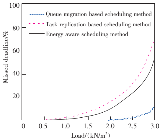
图 6 3 种方法截止期错失率对比分析
