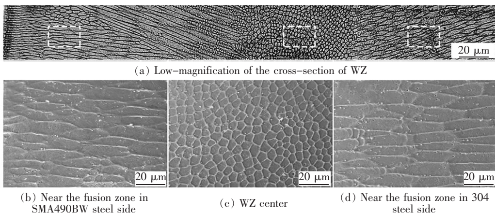
图 1 CrMnFeCoNi 为焊缝填充材料焊接 SM490BW 与 304 不锈钢异种金属焊接区微观结构 [53]
