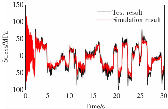
图7 中梁中部焊缝动态应力时域结果对比
