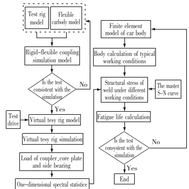
图2 主S-N曲线法的虚拟试验评估流程
