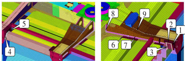
图 3 车体有限元模型
