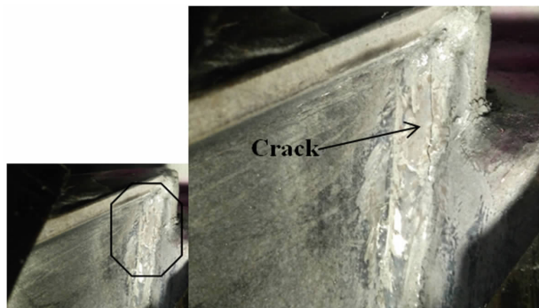
图 11 疲劳裂纹
