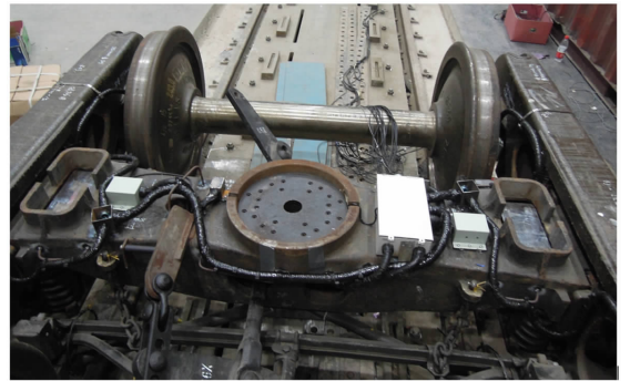
图9 测力摇枕
