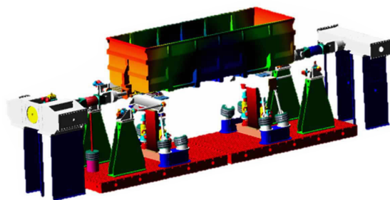
图 1 试验台架的仿真模型
