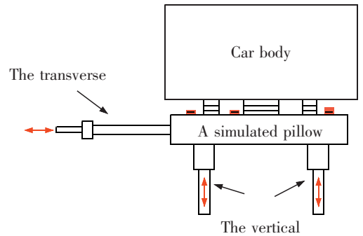
图8 试验台架的简图
