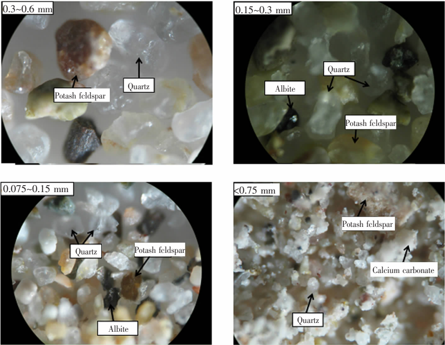
图 6 白色砒砂岩不同粒度的光学显微图片 (100 倍) Fig.6 Optical micrograph of different granularity white Pisha sandstone
