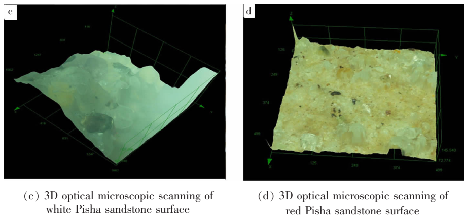
图 9 砒砂岩的光学显微分析 Fig.9 Optical microscope images of Pisha sandstone
