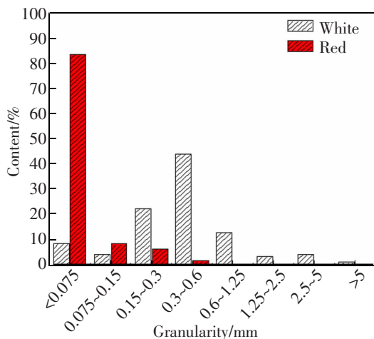
图 1 砒砂岩的粒度分布范围
