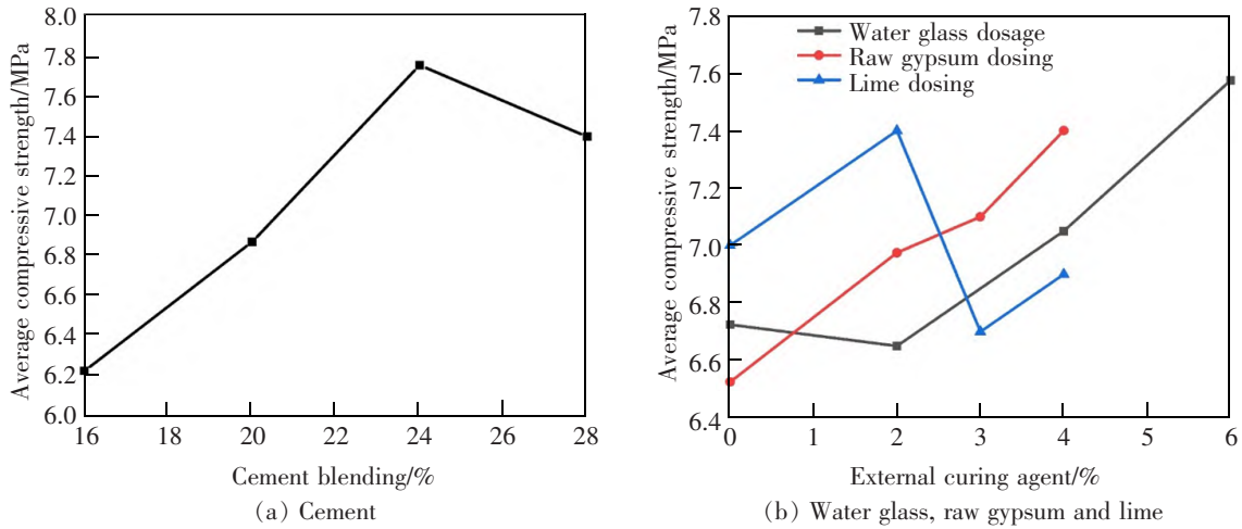
图 3 28 d 各因素的实际掺量与抗压强度的关系
