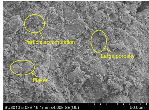
图4 粉质黏土原状土的SEM图像
