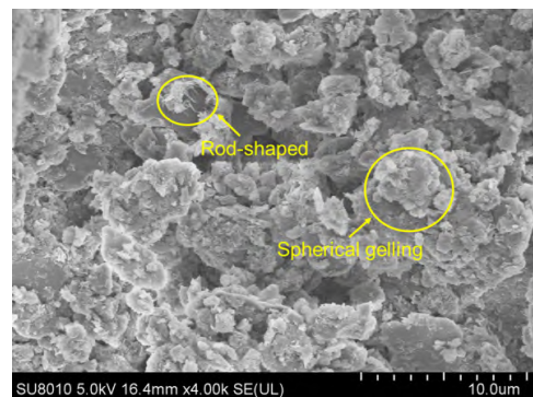
图5 正交试验最优配比组的SEM图像
