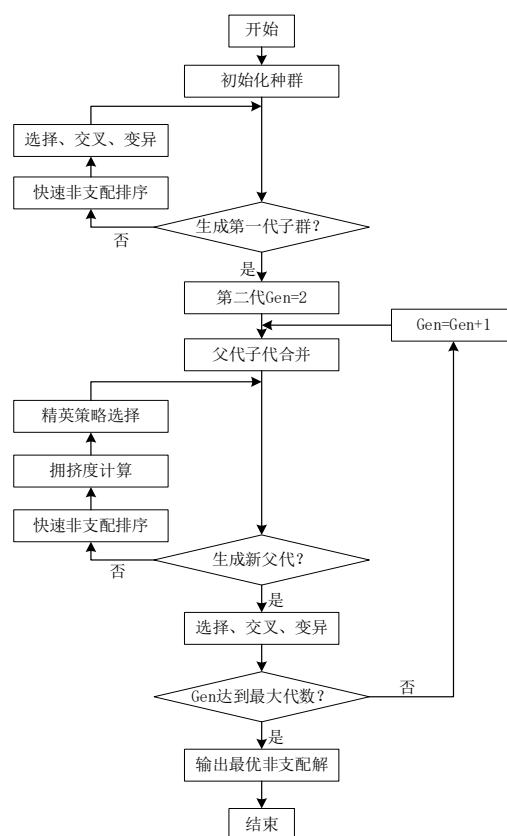
图 1 非支配排序遗传算法流程图
