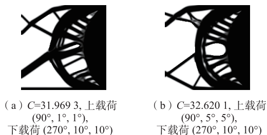
图4 上下载荷不同的扰动范围
