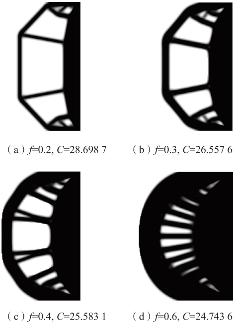
图2 不同体积分数下的拓扑构型
