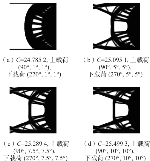
图3 不同扰动范围下的拓扑构型
